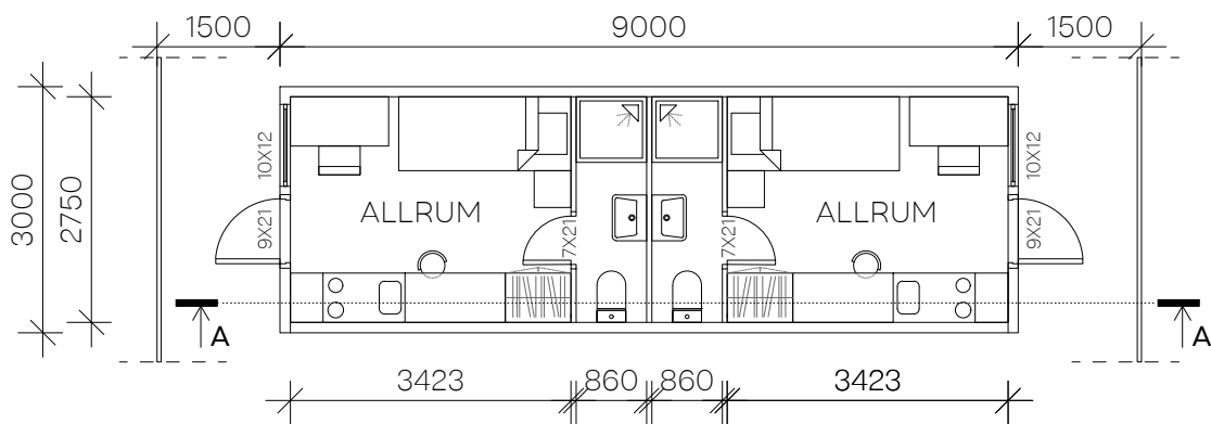
BOTTENVÅNING/ B16 (B15, B17, B18, B19)
