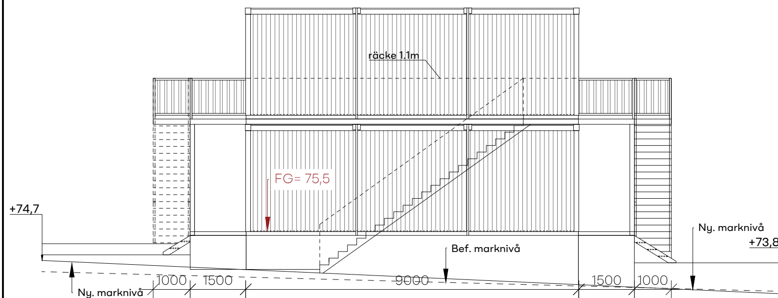
FASAD MOT SYD ÖST/ B16 (B15, B17, B18, B19)
