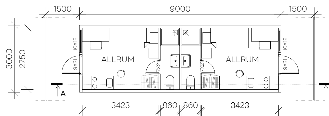
BOTTENVÅNING/ B25 (B20, B21, B22, B23, B24)
