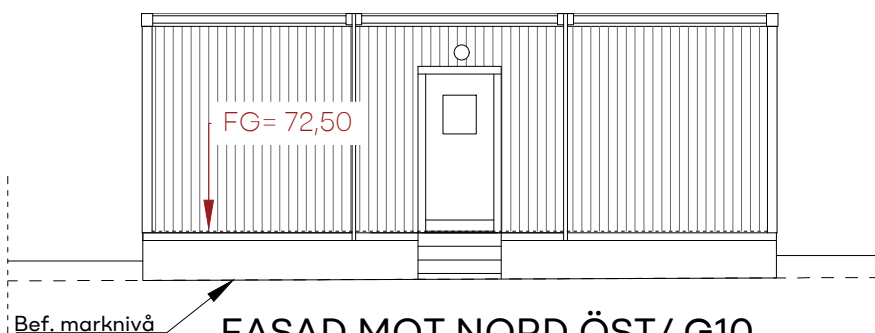
FASAD MOT NORD ÖST/ G10 ( G1, G2, G3 ,G4, G5, G6, G7, G8, G9) 1:100
