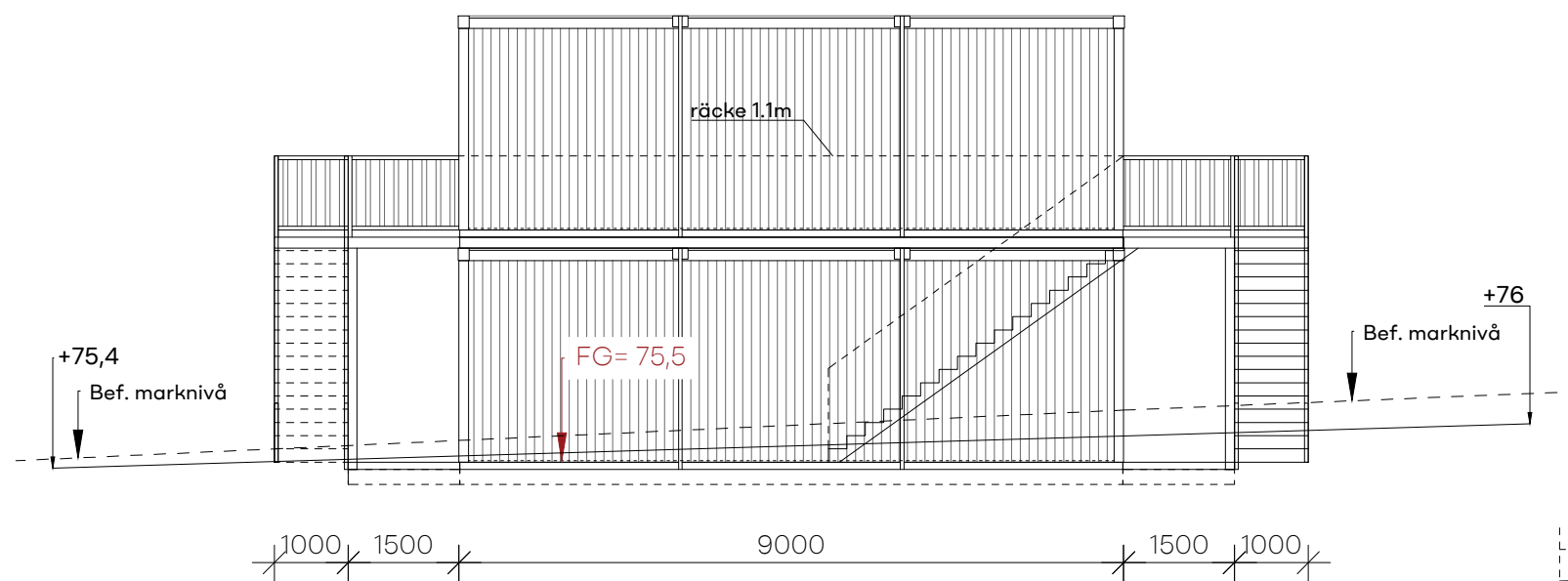
FASAD MOT NORD VÄST/ B16 (B15, B17, B18, B19)
