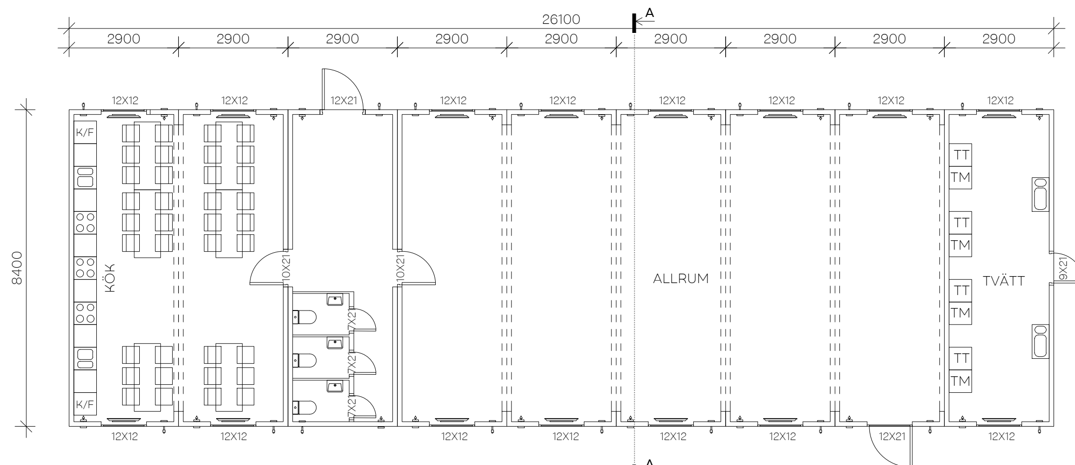
GEMENSAMMA UTRYMMEN - BOTTENVÅNING/ G10 (G1, G2, G3 ,G4, G5, G6, G7, G8, G9)
