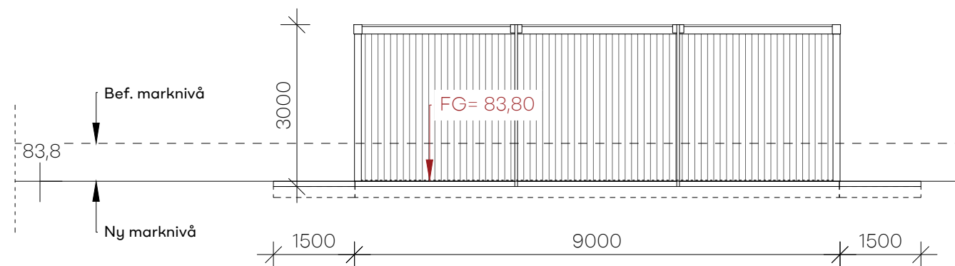
FASAD MOT NORD VÄST/ B3 (B1, B2, B4, B5, B6, B7, B8, B9, B10, B11, B12, B13, B14)
