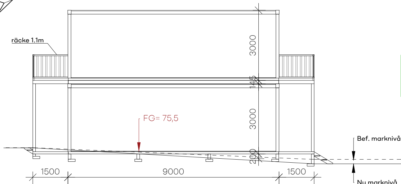
SEKTION A-A/ B16
