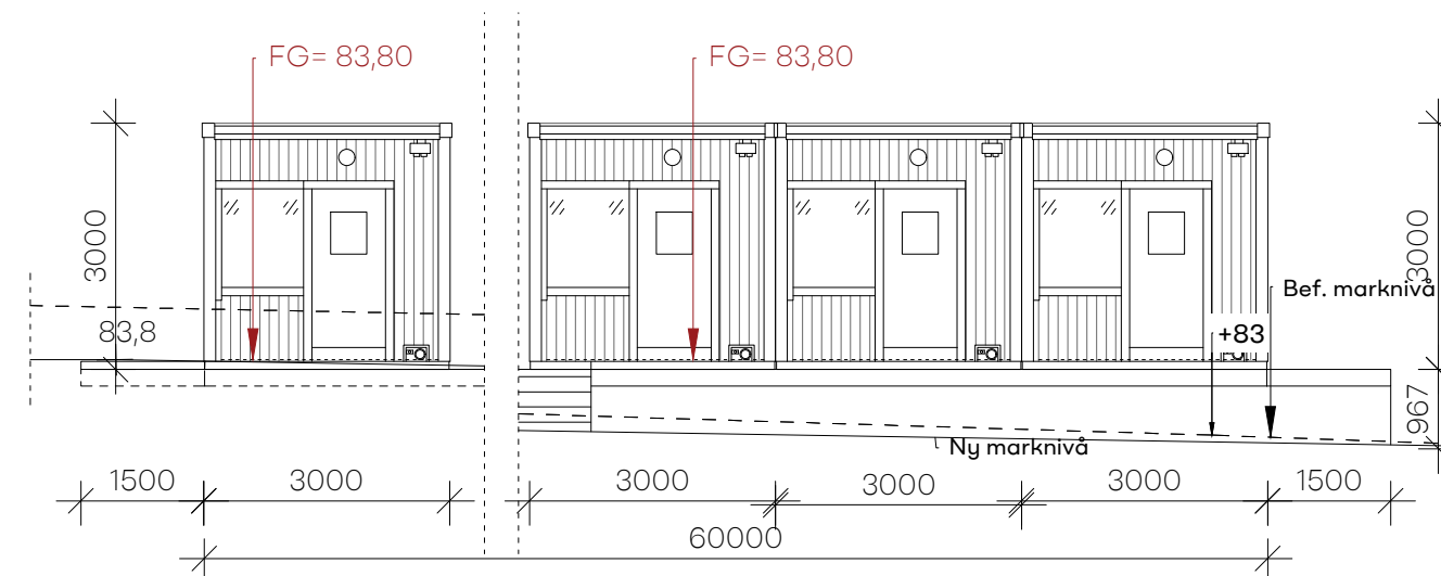
FASAD MOT SYD VÄST/ B3 (B1, B2, B4, B5, B6, B7, B8, B9, B10, B11, B12, B13, B14)
