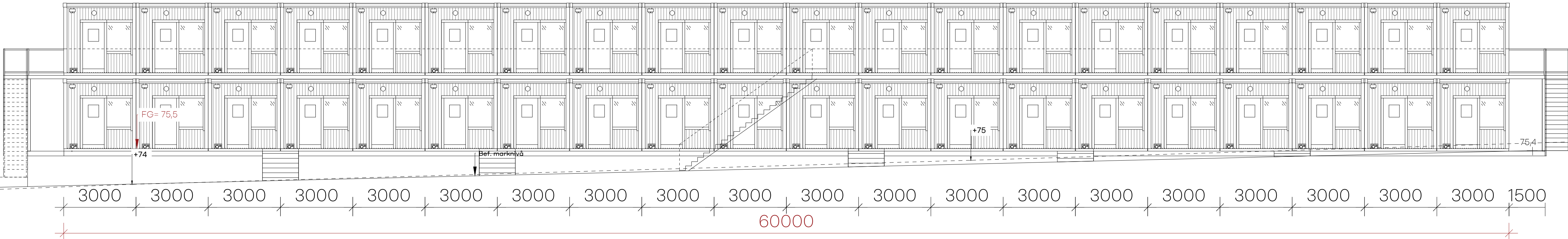
FASAD MOT NORD ÖST/ B16 (B15, B17, B18, B19) 1:100
