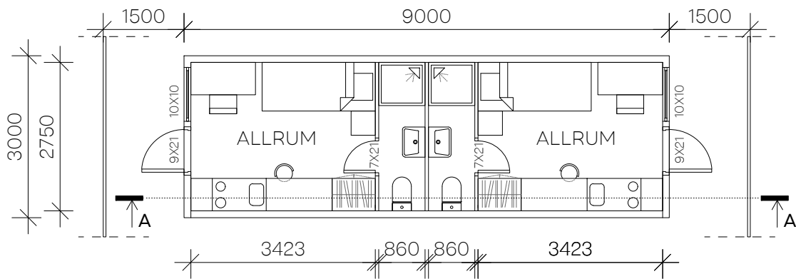
ÖVRE PLAN/ B16 (B15, B17, B18, B19)
