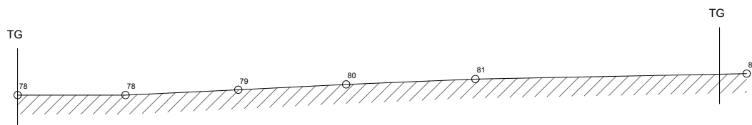
BEF. SEKTION C-C 1:1000
