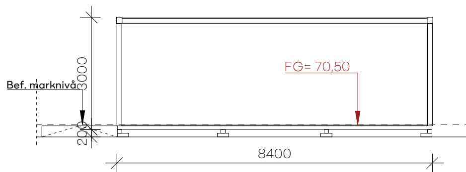
SEKTION A-A/ R1
