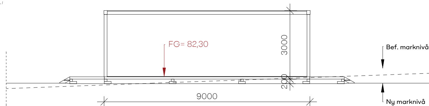
SEKTION A-A/ B25 (B20, B21, B22, B23, B24)
