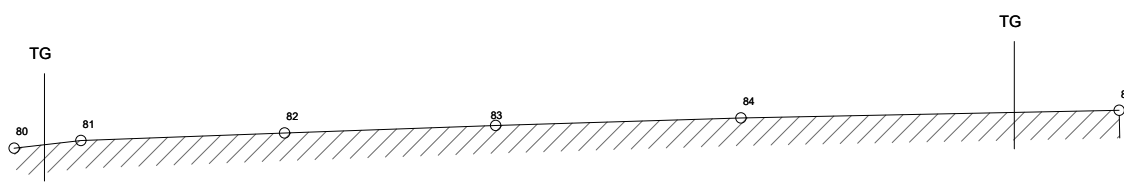
BEF. SEKTION A-A 1:1000
