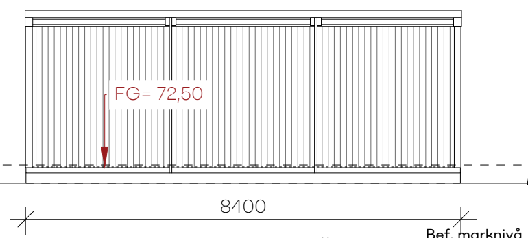
FASAD MOT SYD VÄST/ G10 ( G1, G2, G3 ,G4, G5, G6, G7, G8, G9) 1:100
