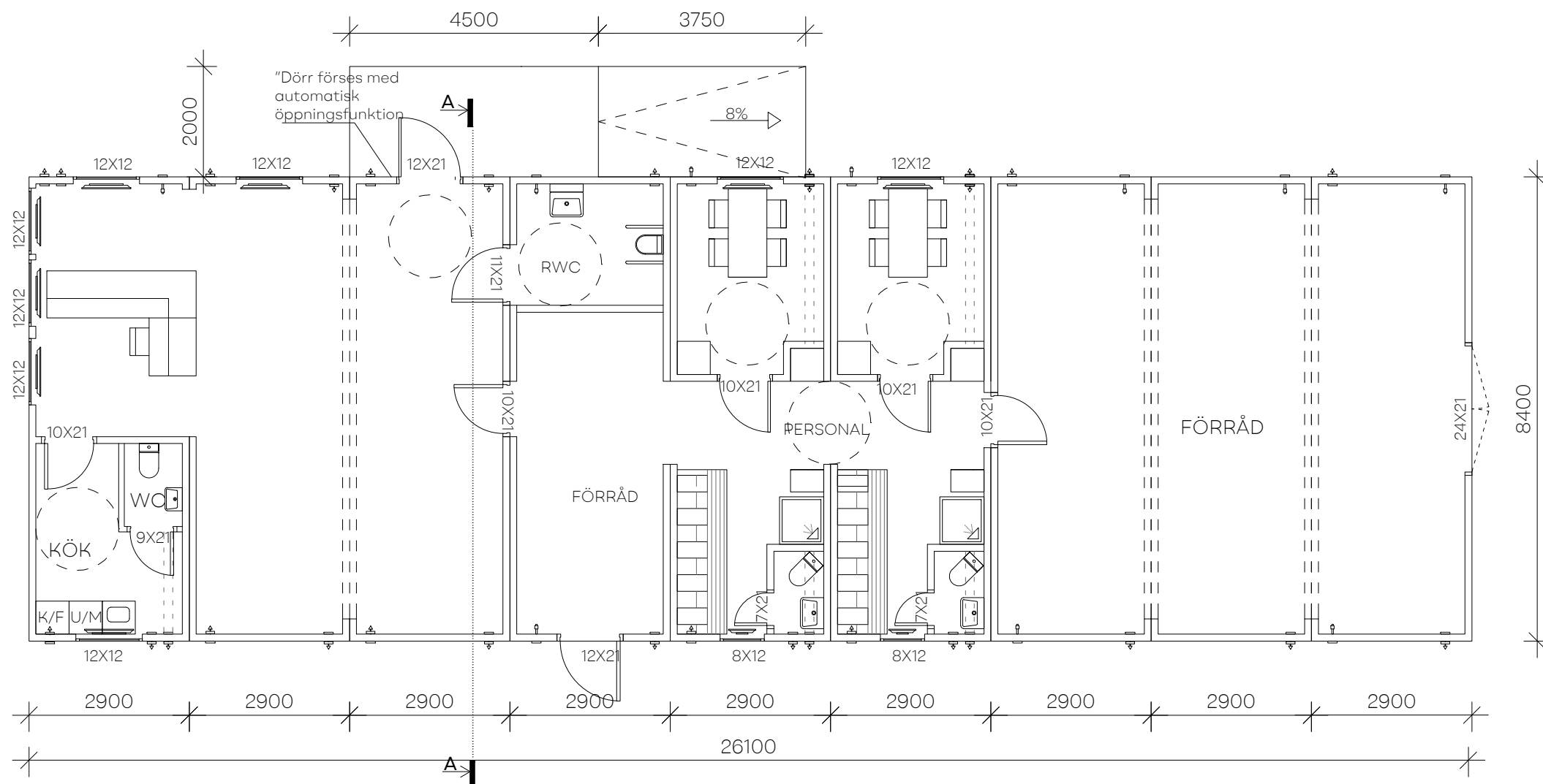
ADMINISTRATION - BOTTENVÅNING/ R1
