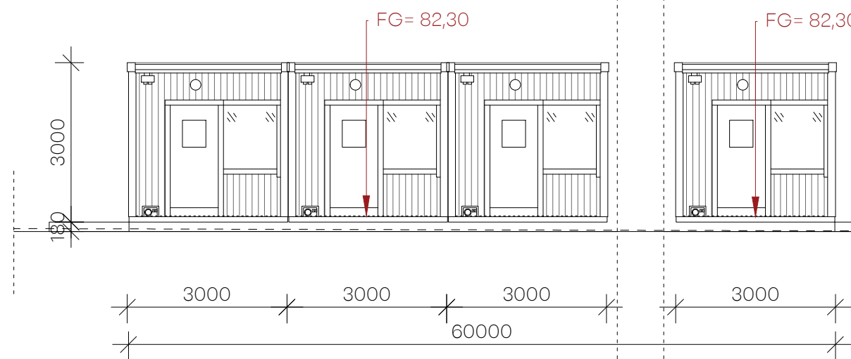
FASAD MOT NORD VÄST/ B25 (B20, B21, B22, B23, B24)
