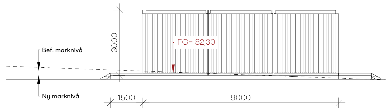
FASAD MOT SYD VÄST/ B25 (B20, B21, B22, B23, B24)
