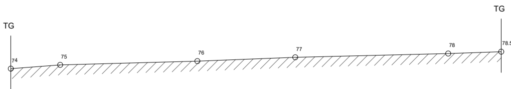
BEF. SEKTION D-D 1:1000
