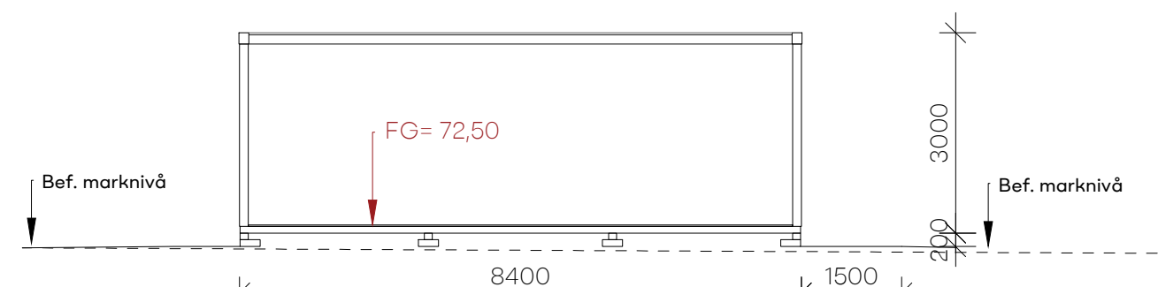
SEKTION A-A/ G10 (G1, G2, G3 ,G4, G5, G6, G7, G8, G9)
