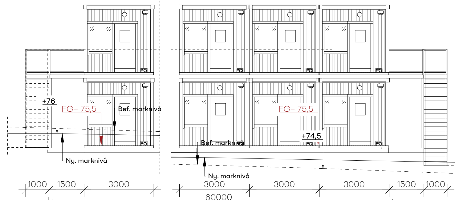
FASAD MOT SYD VÄST/ B16 (B15, B17, B18, B19)
