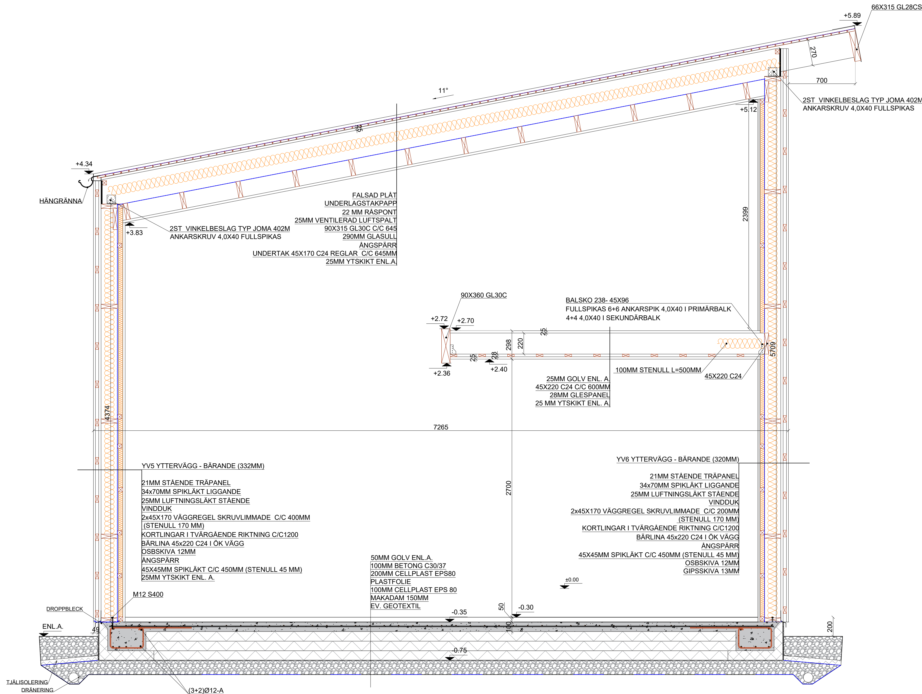
Sektion A-A 1:20
