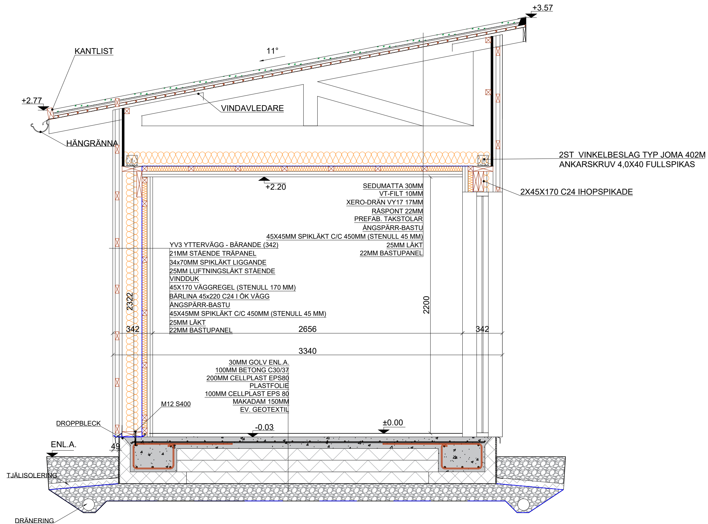
Sektion D-D 1:20
