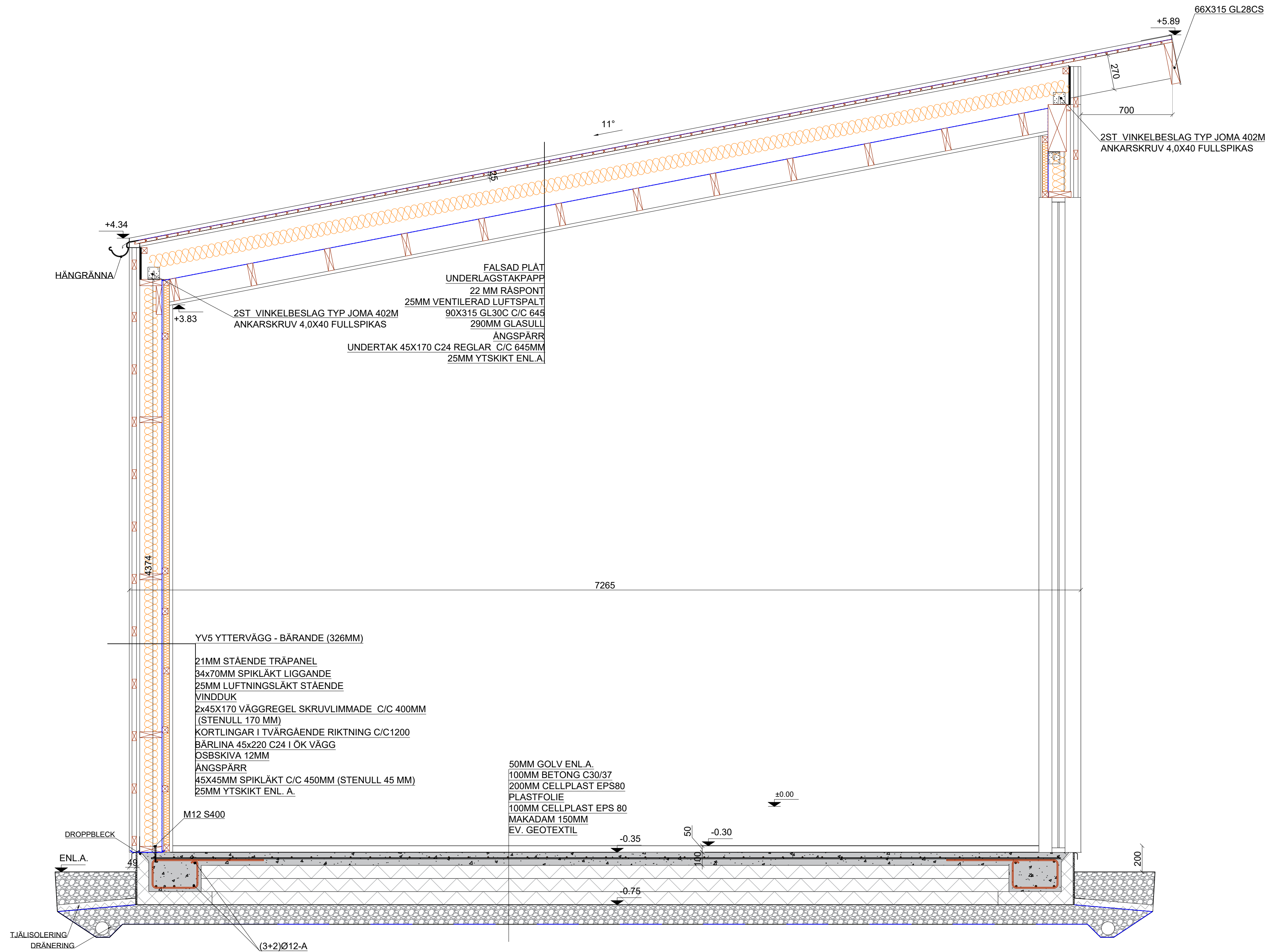
Sektion A-A 1:20
